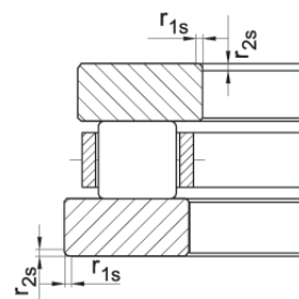
Axialzylinderrollenlager
