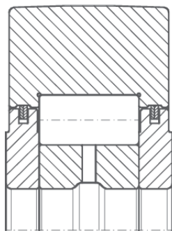
Stützrolle/Carrier roller
