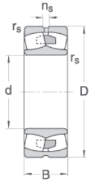
Zylindrische Bohrung/ cylindrical bore
