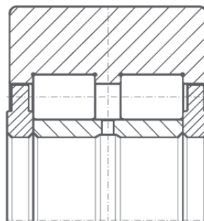
Mehrreihige vollrollige Zylinderrollenlager Cageless multirow cylindrical roller bearings
