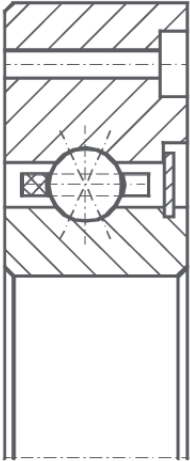
Vierpunktlager für die Textilindustrie Four point bearing for textile machines
