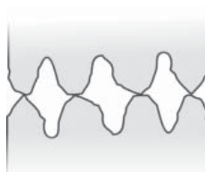
Grenzfall der Berührung der Metalloberflächen \kappa = 1
