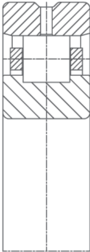
Lager für Rohrverleimmaschinen mit minimiertem Reibquerschnitt und Schmierbohrungen auf der Laufbahn Bearing for tube stranding machines with minimized friction cross section and lube bores at the race
