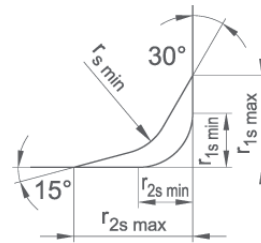
Beispiel: Innenring eines Rillenkugellagers mit symmetrischem Querschnitt
